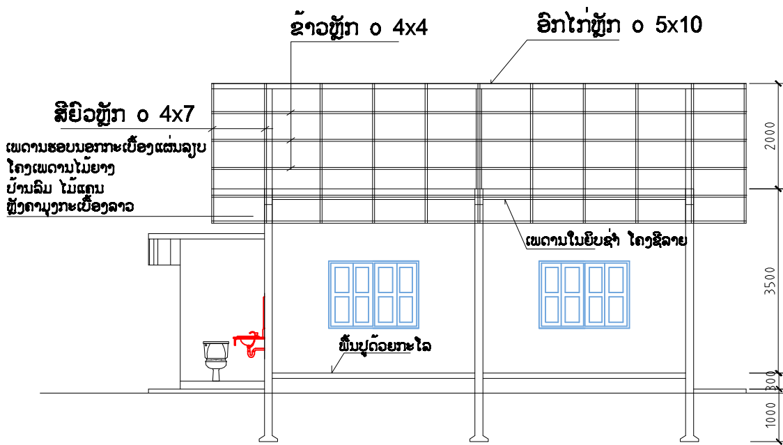
ຮູບຕັດ 1-1 ມ:1/100
