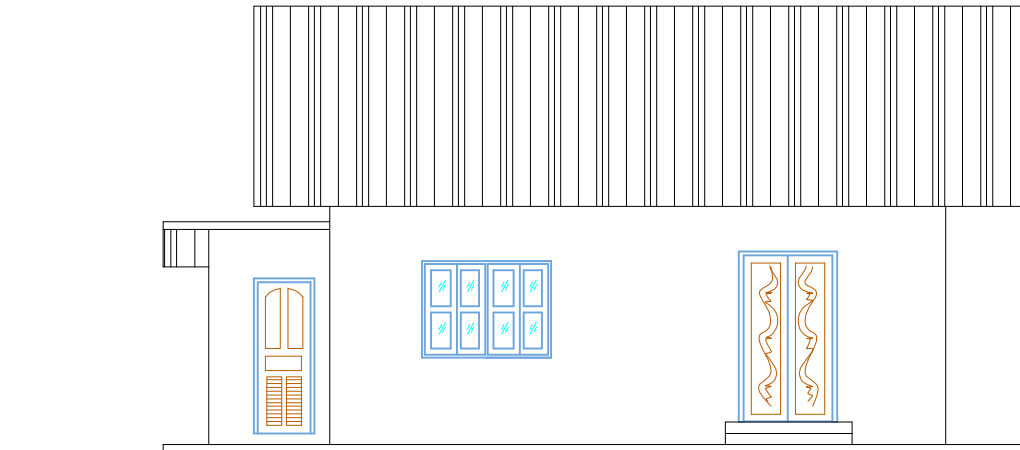
ຮູບດ້ານໜ້າ ມ:1/100
